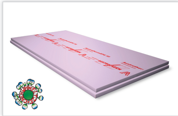
Austrotherm XPS TOP (polistyren ekstrudowany) – nowa generacja różnorodnych płyt z polistyrenu ekstrudowanego, w produkcji których zamiast szkodliwych dla atmosfery gazów używa się wyłącznie dwutlenku węgla. To termoizolacja spełniająca wszystkie wymagania stawiane ociepleniu w ekstremalnych warunkach pracy i pod różnymi obciążeniami. Ich cechą charakterystyczną jest bardzo duża wytrzymałość na ściskanie.
